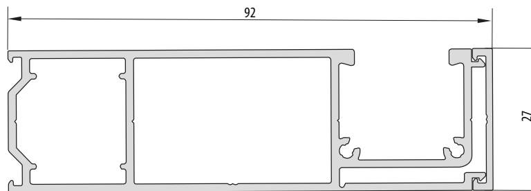
Monoblock-Führungsschiene
