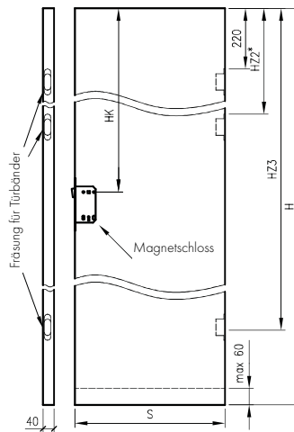
Türflügel ohne Falz: Standard 10, Modern, Plus
