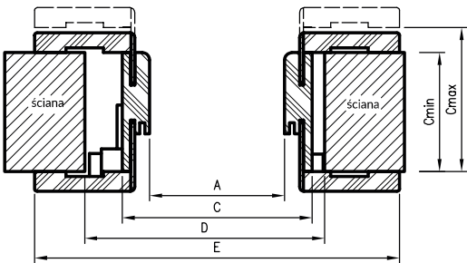
Horizontalschnitt ORB
