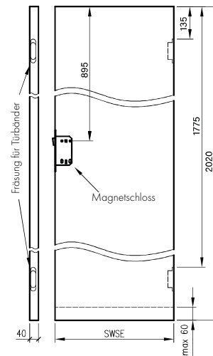
Türflügel ohne Falz Sara Eco 2 im Standard 202X
