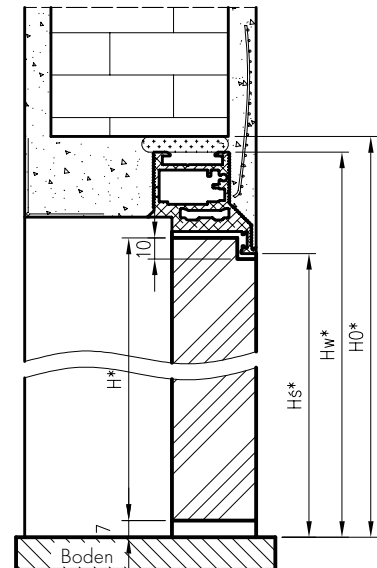
Vertikalschnitt Sara Eco 2 Tür mit Falz nach außen öffnend
