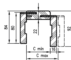
Schnitt TUN-Profil mit Winkel. T80
