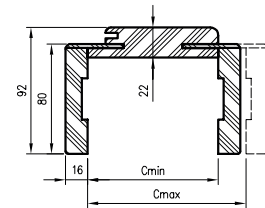
Schnitt OR/ORC mit Winkel T80
