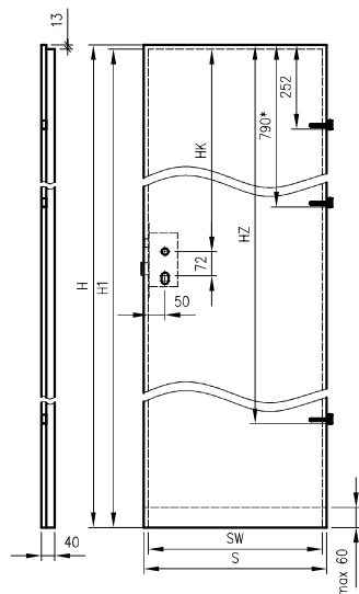
Türflügel ohne Falz: Standard 10, Modern, Plus
