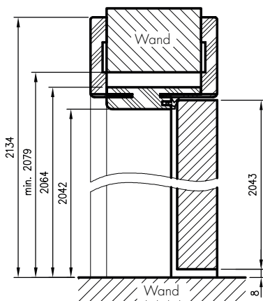
Vertikalschnitt der Türflügel ohne Falz im ORB
