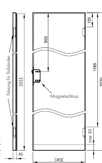
Türflügel mit Falz Sara Eco 2 im Standard 202X
