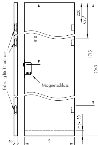
Türflügel ohne Falz
