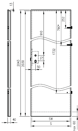
Türflügel ohne Falz
