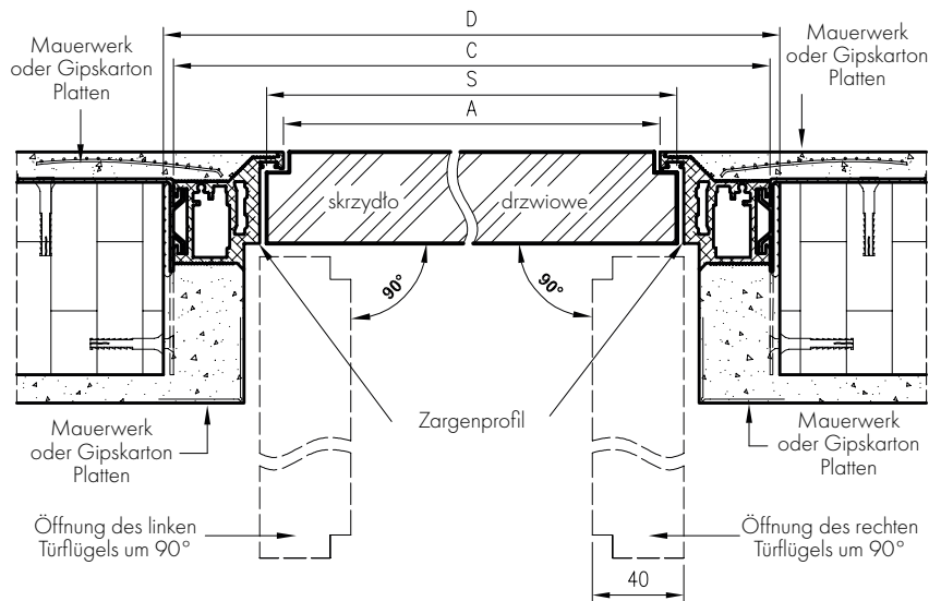
Querschnitt Sara Eco 2 Tür mit Falz nach innen öffnend
