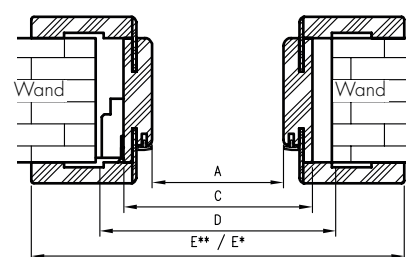
Horizontalschnitt OR/ORC
