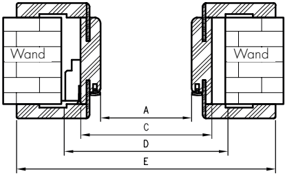
Horizontalschnitt OR
