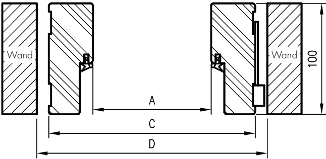
Horizontalschnitt OPB
