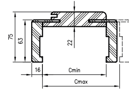
Schnitt OR/ORC mit Winkel T63
