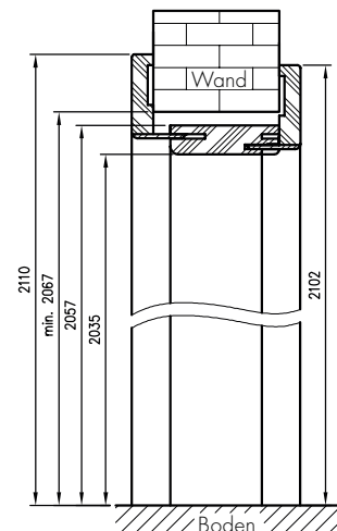
Vertikalschnitt des verstellbaren Tunnels mit Winkel. T63
