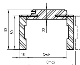
Schnitt OR/ORC-Profil mit Winkel T80
