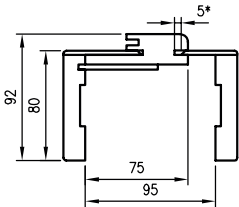
Schnitt ORB 075
