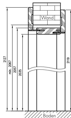
Vertikalschnitt des verstellbaren Tunnels mit Winkel. T80
