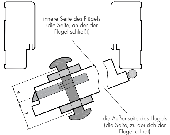
Abb. Auswahl der Größe des Zylinders mit Drehknopf
