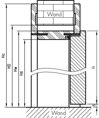
Vertikalschnitt OR
