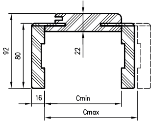
Horizontalschnitt OR
