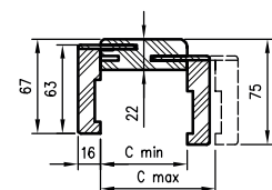
Schnitt TUN-Profil mit Winkel. T63
