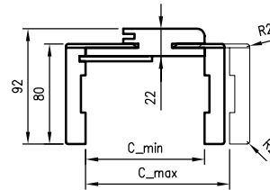
Schnitt ORB 095-300
