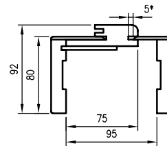
Schnitt ORB 075
