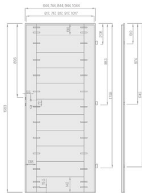
Flügel mit Falz
