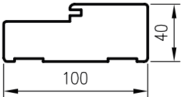
OPB Profil
