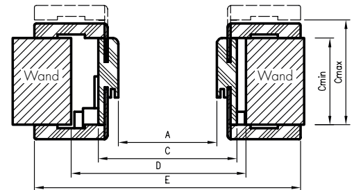
Horizontalschnitt ORB
