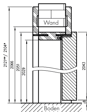
Vertikalschnitt eines Türflügels mit Falz mit OR
