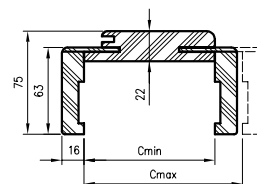
Schnitt OR/ORC-Profil mit Winkel T63
