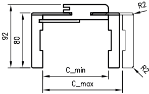
Schnitt ORB 075
